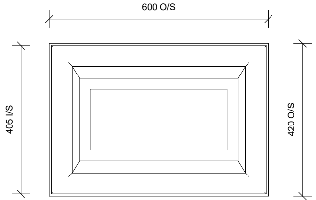
TOP 1 : 10
