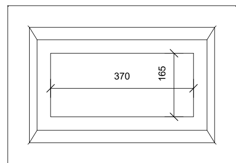
BOTTOM 1 : 10
