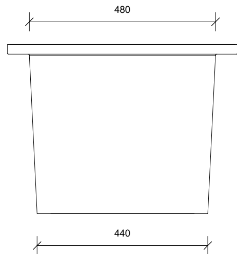
FRONT 1 : 10
